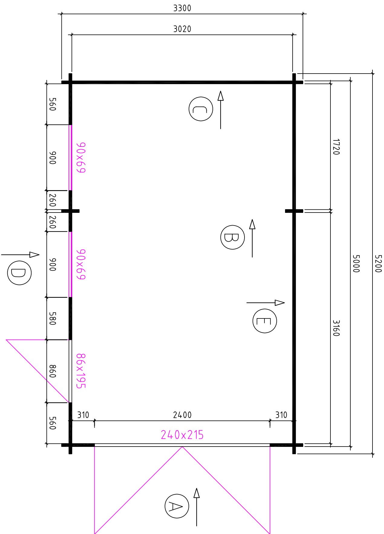
Grundplan
